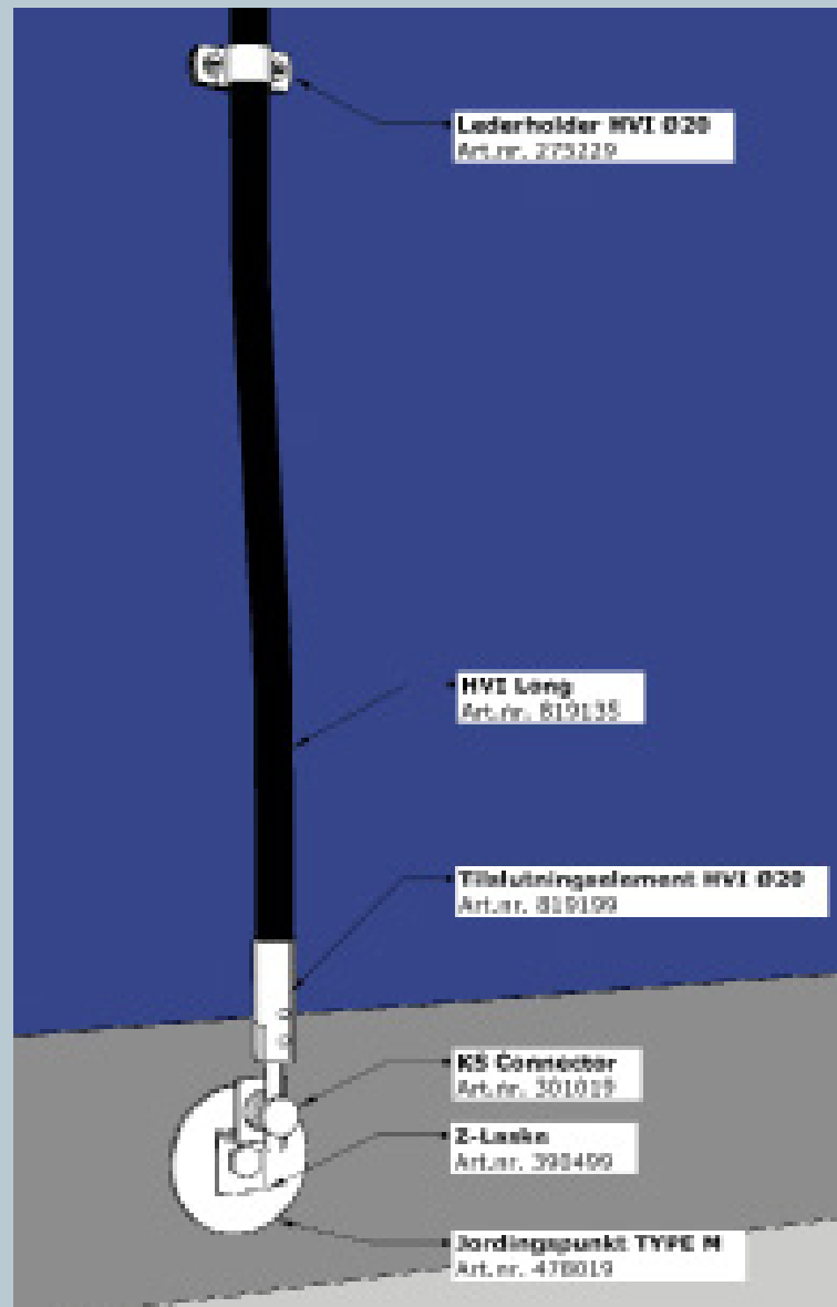
Detaljtegning Tilslutning til fundamentsjord
