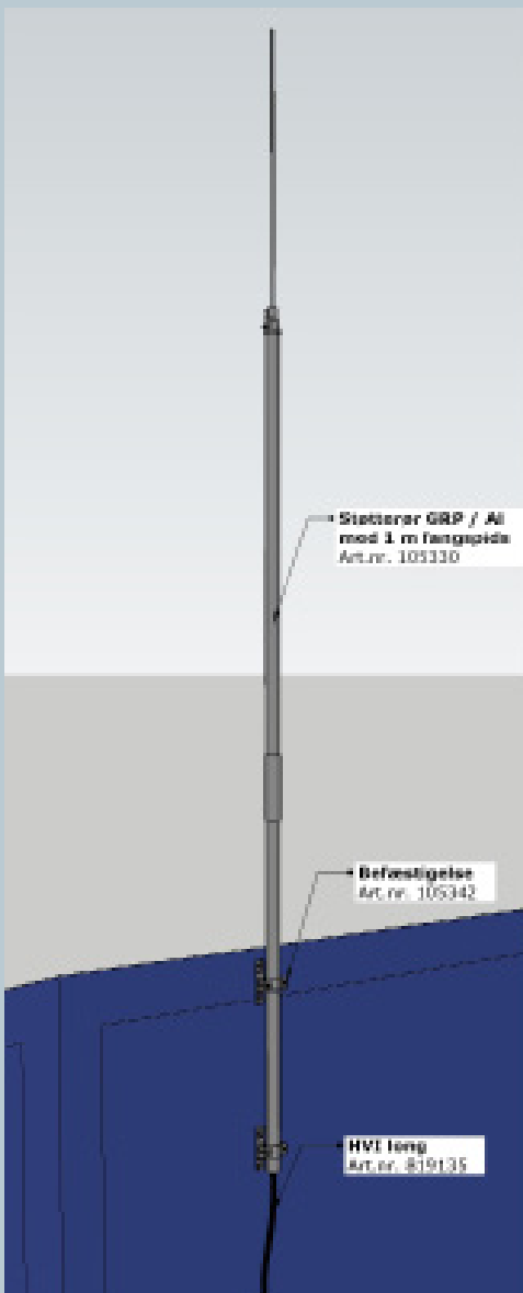
Detaljtegning Fangstang
