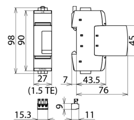
Målskitse DG SE 1000 VA WE FM
