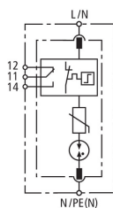
Elektrisk opbygning DG SE 1000 VA WE FM
